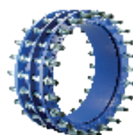
Серия 873 Трехфланцевая демонтажная вставка DN40-2600 PN10/16/25 Высокопрочный чугун
